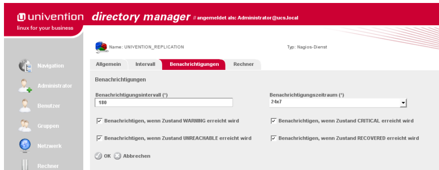
Abbildung 3: Karteikarte "Benachrichtigungen" eines Nagios:Dienst-Objektes
