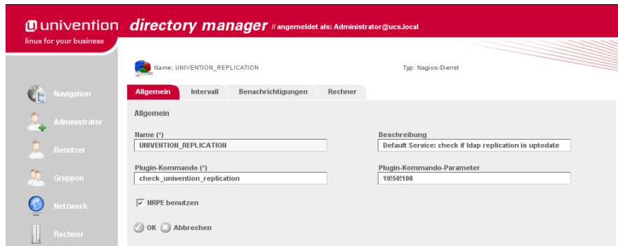
Abbildung 5: Beispielhafte Verwendung des check_univention_replication-Kommandos
